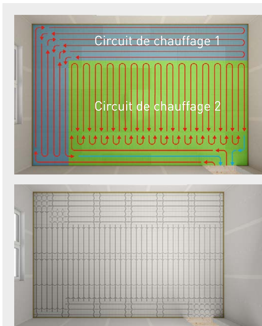
Schéma d'installation avec deux boucles de chauffage
