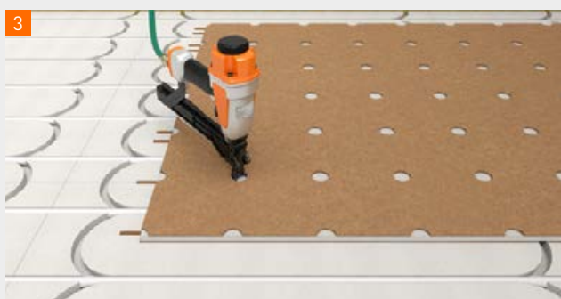
Placez la plaque supérieure et fixez-la mécaniquement au moyen de vis ou d'agrafes expansives en vous servant du gabarit.
