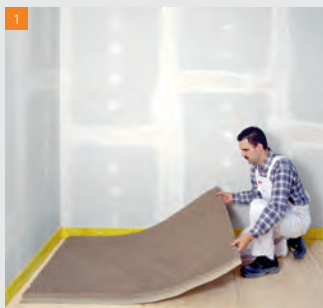
1 Poser les Plaques de sol en nids-d'abeilles fermacell
