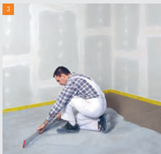
3 Aplanir les granules pour nid-d'abeilles fermacell
