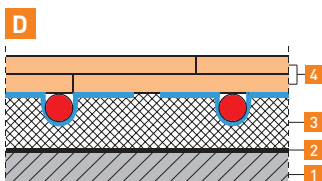
Plaque de sol fermacell (2 E 22) sur système de chauffage au sol à eau (dessous)
