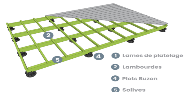
Double structure en solives + lambourdes
