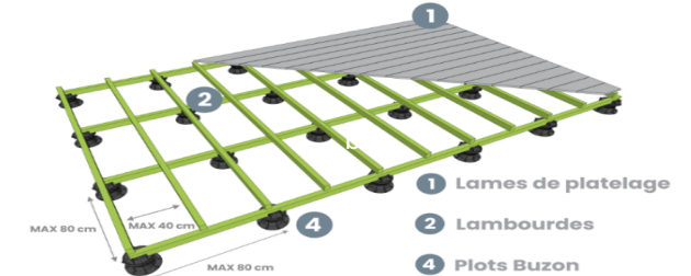
Double structure en lambourdes
