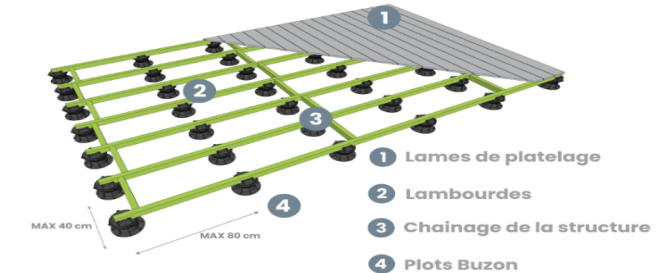
Simple structure en lambourdes
