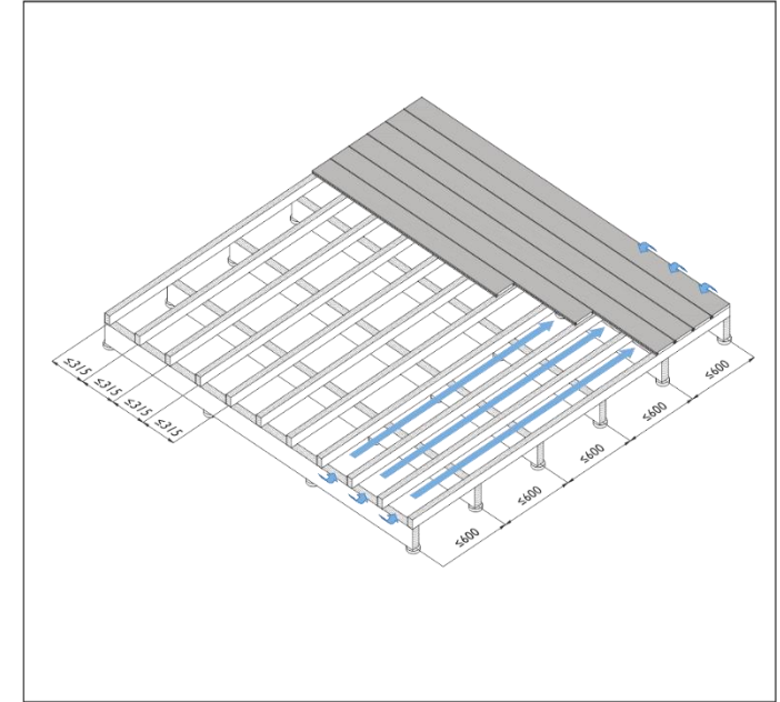
Les lames Cedral Terrasse reposent sur un double lattage.
