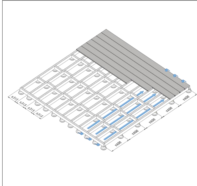
On prévoit des chaînages de structure tous les 60 cm (les lambourdes ne peuvent pas être fixées dans le sol).
