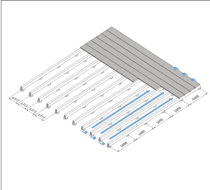
Les lames de Cedral Terrasse sont fixées sur un simple lattage.
